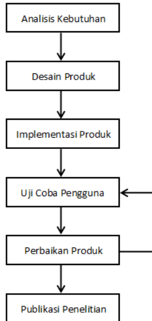
Gambar 3.2. Prosedur Pengembangan
